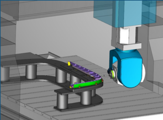
VERICUT SANAL CNC TEZGAHI ÜZERİNDE SİMÜLASYON
